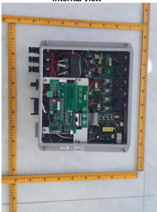
Invólucro - Visão interna Internal view
