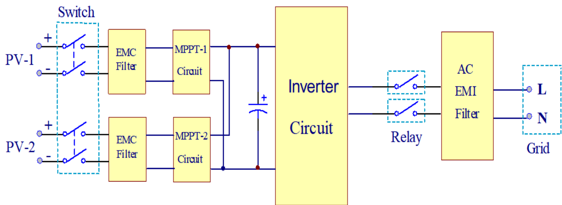
Diagrama de bloco: Block Diagram:
