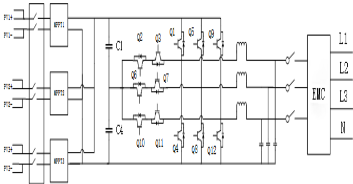
Diagrama de bloco: Block Diagram:
