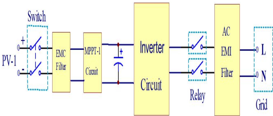
Diagrama de bloco: Block Diagram:
